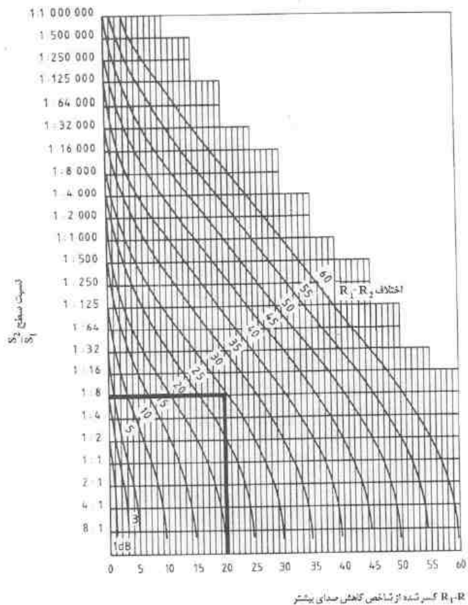
شکل پ-۱-۲: نمودار تخمین شاخص کاهش صدای جداکننده مرکب
