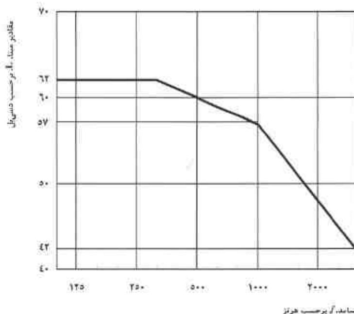
شکل ۱۸-۱-۳: نمودار مقادیر منهای صدای کوبه‌ای، در بندهای یک‌سوم هتگامی
