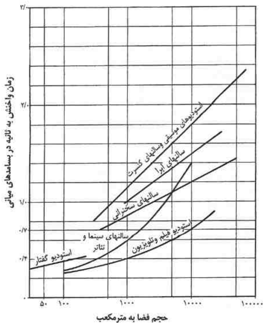
شکل ۲-۱۸-۷-۱: نمودار زمان واختم بهینه در فضاهای مختلف
