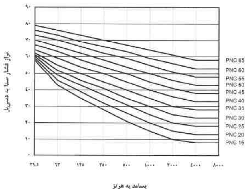
شکل ۱۸-۱-۳-۵: نمودارهای برسنج ترجیحی نوفه PNC
