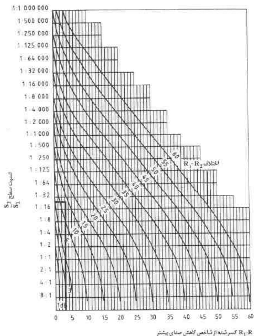
شکل ب-۱-۳: نمودار تخمین شاخص کاهش صدای جداکننده مرکب
