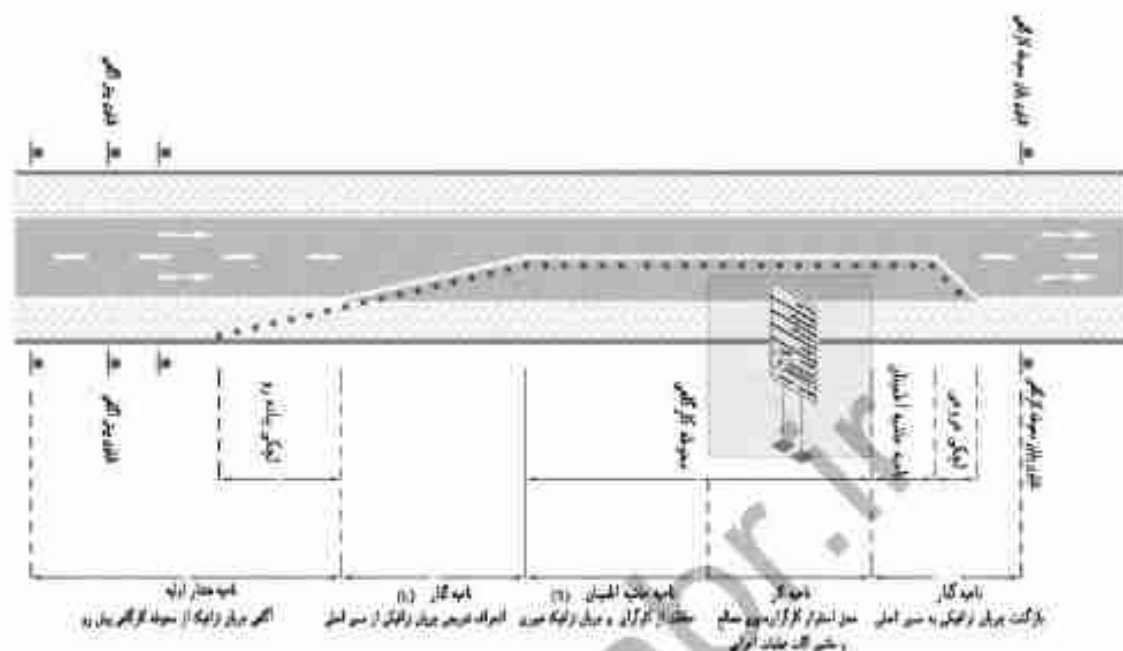
شکل ۲۳-۱-۱ محدوده حفاظت از عملیات کارگاهی
