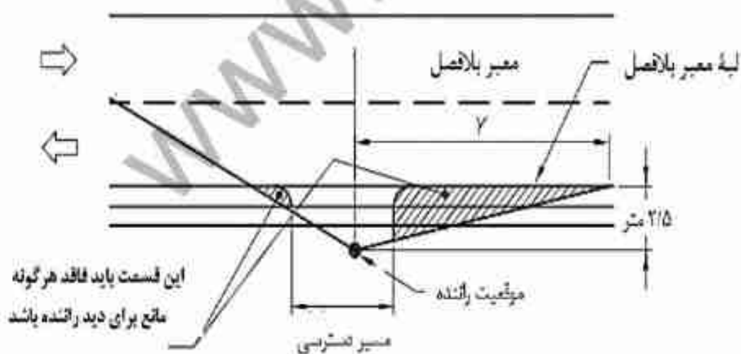
شکل ۲۳-۴-۱-۲ مسافت دید مسیر دسترسی به پارکینگ
