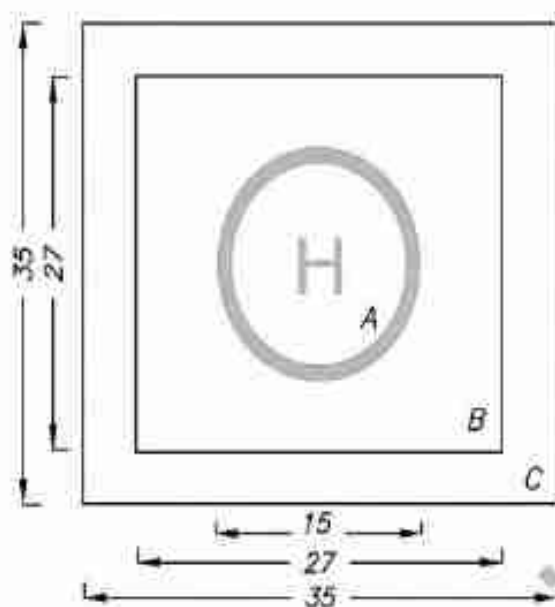
شکل ۳۳-۴-۹ ابعاد محل فرود بال گرد مستطیلی
